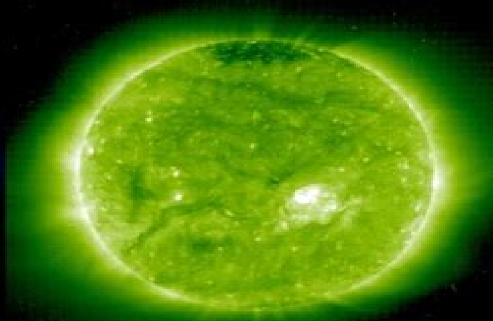
Fe XII, 195 Angstroms
